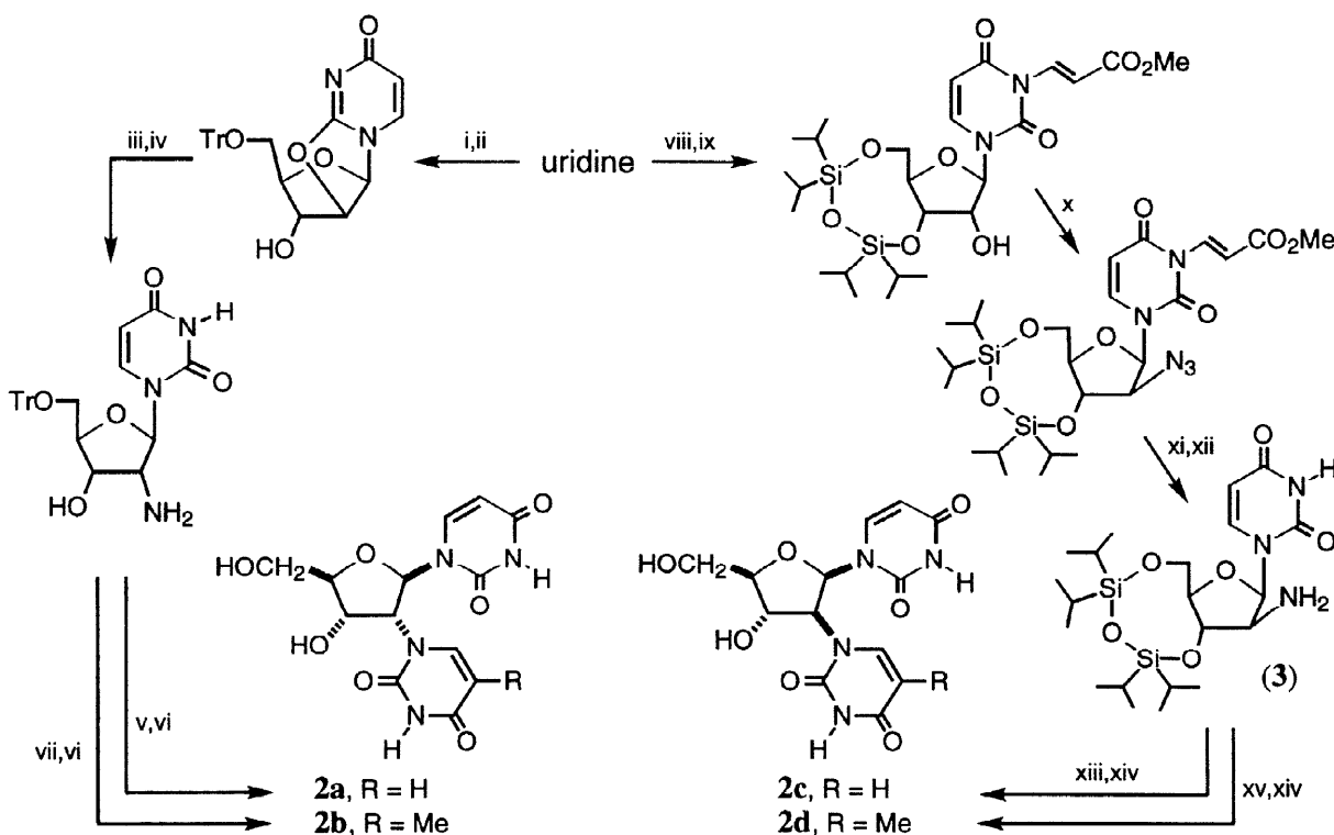
Scheme 2. i, TrCl, py, 120 °C, 2 h, 95%; ii, \text{Im}_2\text{C}=\text{S} , toluene, 110 °C, 30 min, 80%; iii, \text{Me}_3\text{SiN}_3 , LiF, DMF/TMEDA, 110 °C, 48 h, 60%; iv, \text{SnCl}_2/\text{PhSH}/\text{Et}_3\text{N} , \text{CH}_3\text{CN} , rt, 30 min, 95%, or \text{H}_2 , Pd/C, MeOH, rt, 1 h, 95%; v, \text{EtOCH}=\text{CH}-\text{CO}-\text{N}=\text{C}=\text{O} (1.2), \text{C}_6\text{H}_6/\text{DMF} 1:1, rt, 3 h, 85%; vi, 1 M \text{H}_2\text{SO}_4/\text{dioxan} , \Delta , overnight, 80–90%; vii, \text{MeOCH}=\text{CMe}-\text{CO}-\text{N}=\text{C}=\text{O} (1.2), \text{C}_6\text{H}_6/\text{DMF} , rt, 3 h, 85%; viii, \text{ClSiPr}_2\text{OSiPr}_2\text{Cl} (1.05), py, rt, overn., 95%; ix, \text{HC}\equiv\text{C}-\text{COOMe} (1.0), DMAP (0.3), \text{CH}_3\text{CN}/\text{CH}_2\text{Cl}_2 4:1, rt, 40 min, 88%; x, \text{Ph}_3\text{P}/\text{DEAD}/(\text{PhO})_2\text{PON}_3 (3.0), THF, 0–20 °C, overnight, 68%; xi, pyrrolidine, \text{CH}_3\text{CN} , rt, 3 h, 98%; xii, \text{H}_2 , Pd/C, MeOH, rt, 3 h, then MeOH, 40 °C, 12 h, 65%; xiii, \text{EtOCH}=\text{CHCO}-\text{NCO} (2.0), \text{C}_6\text{H}_6/\text{DMF} , rt, 5 h, 72%; xiv, 1 M \text{H}_2\text{SO}_4/\text{dioxan} , \Delta , 5 h, 70–75%; xv, \text{MeOCH}=\text{CMeCO}-\text{NCO} (2.0), \text{C}_6\text{H}_6/\text{DMF} , rt, 5 h, 70%.
