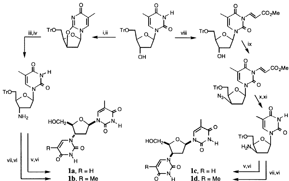
Scheme 1. i, \text{MeSO}_2\text{Cl} , py, 0 °C, 15 h, 95%; ii, \text{K}^+ phthalimide ^- , DMF/ \text{H}_2\text{O} , 90 °C, 3 h, 85%; iii, \text{NaN}_3 , DMF/ \text{H}_2\text{O} , \Delta , 15 h, 80%; iv, \text{SnCl}_2/\text{PhSH}/\text{Et}_3\text{N} (1.5:4.5:4.5), \text{CH}_3\text{CN} , rt, 30 min, 85%; v, \text{EtO}-\text{CH}=\text{CH}-\text{CO}-\text{N}=\text{C}=\text{O} (2.0), \text{C}_6\text{H}_6/\text{DMF} , rt, 2 h, \approx 90\% ; vi, 1 M \text{H}_2\text{SO}_4/\text{dioxan} , \Delta , 4 h, 80–85%; vii, \text{MeO}-\text{CH}=\text{CMe}-\text{CO}-\text{N}=\text{C}=\text{O} (2.0), \text{C}_6\text{H}_6/\text{DMF} , rt, 2 h, 85%; viii, \text{HC}\equiv\text{C}-\text{COOMe} (1.0), DMAP (0.3), \text{CH}_3\text{CN}/\text{CH}_2\text{Cl}_2 , rt, 40 min, 83%; ix, \text{Ph}_3\text{P}/\text{DEAD}/(\text{PhO})_2\text{PON}_3 (3.0), THF, 0–20 °C, 5 h, 97%; x, \text{SnCl}_2/\text{PhSH}/\text{Et}_3\text{N} , \text{CH}_3\text{CN} , rt, 5 h, 75%; xi, pyrrolidine (exc.), \text{CH}_3\text{CN} , rt, 4 h, 94%.
